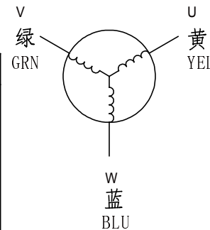
绕组接线图
