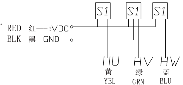
霍尔接线图
