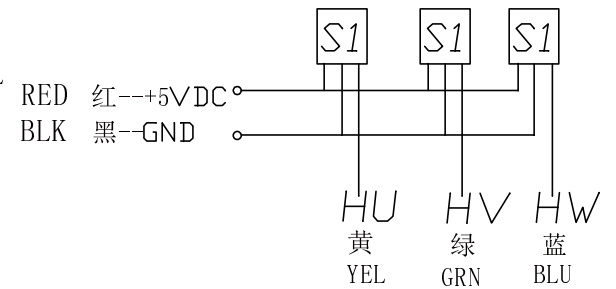
霍尔接线图
