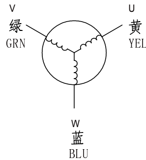
绕组接线图
