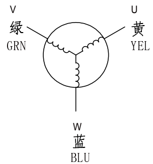
绕组接线图
