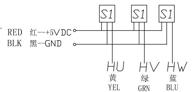
霍尔接线图
